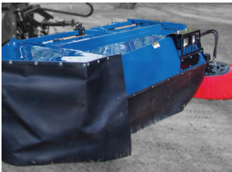
Cabeza de hileradora
